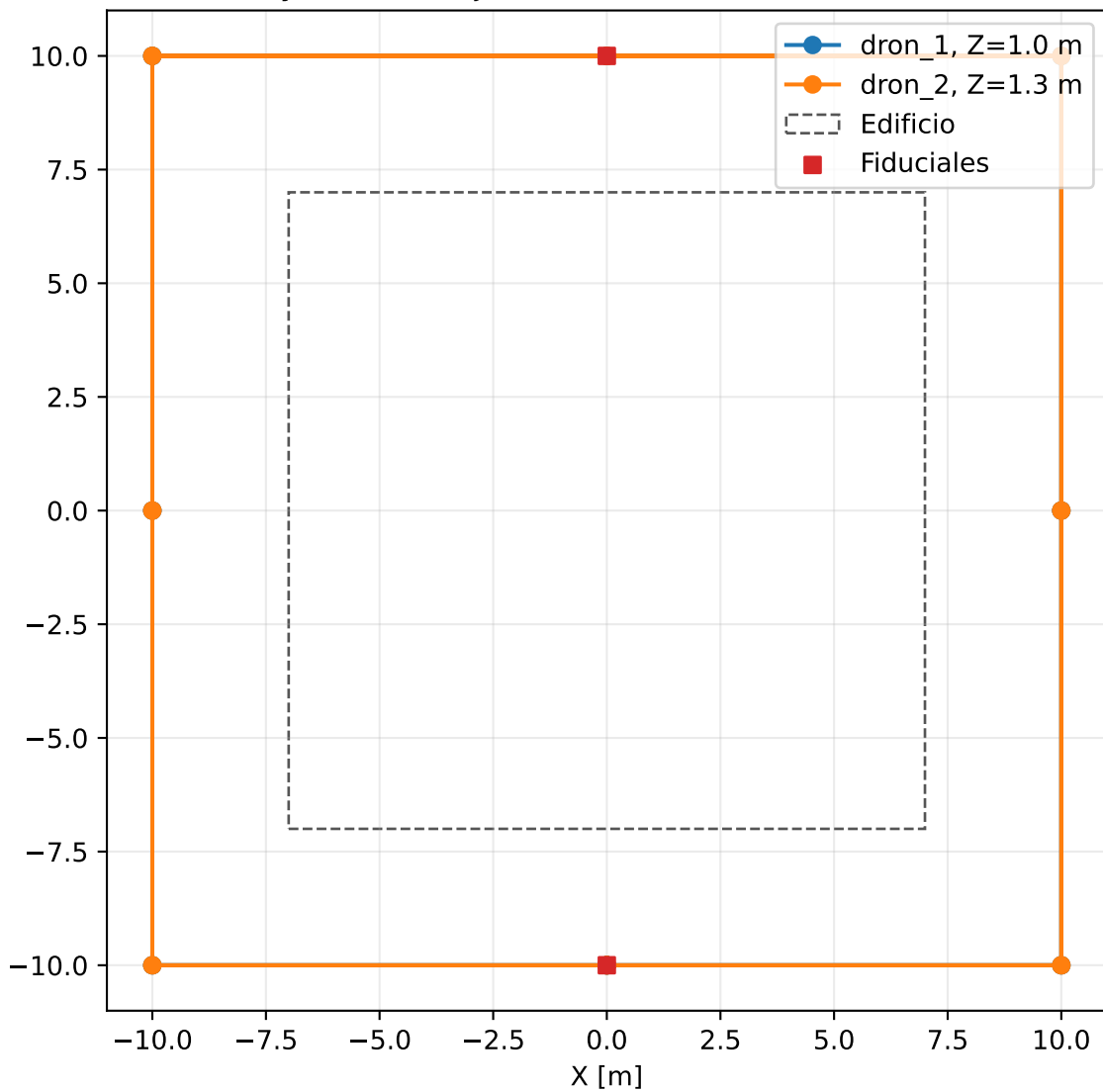
Trayectorias objetivo XY: dos vueltas contrarias
